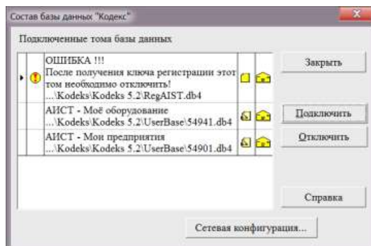
Рис.3.4. Отключить RegAIST.db4.
